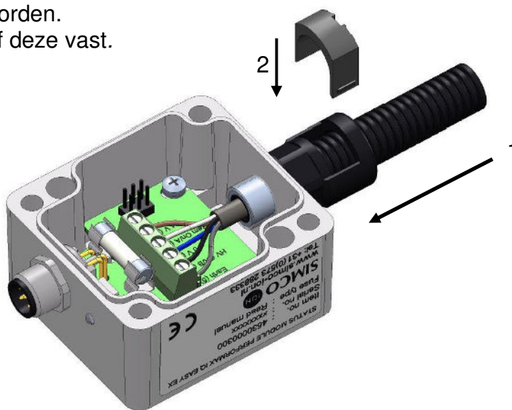
Afbeelding 5.8.2.5: Beschermsslant bevestigen aan wartel
